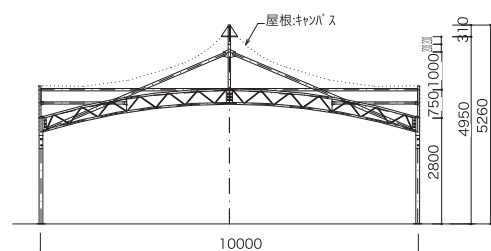
【断面図】
