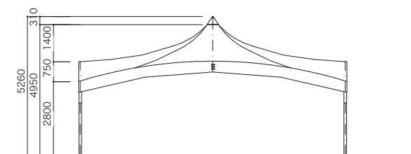
【立面図】
