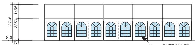
【立面図】
