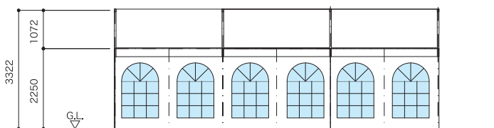
【立面図】
